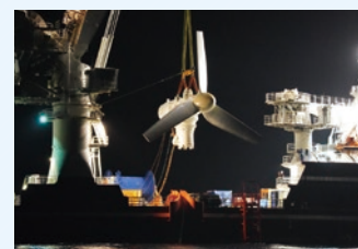
海底への設置作業
